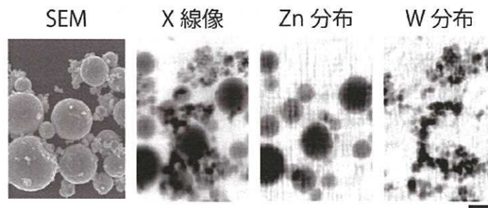
図 2 XAFS イメージングによる元素識別。亜鉛(Zn)粒子とタンゲステン(W)粒子を観察した。 スケールバー:2μm。
